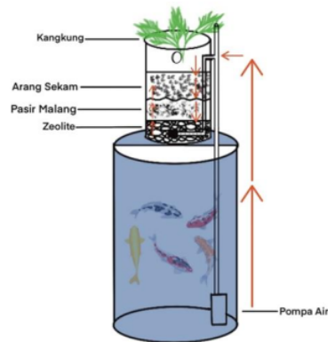
Gambar 1. Vertiqua biofikal filter atas
