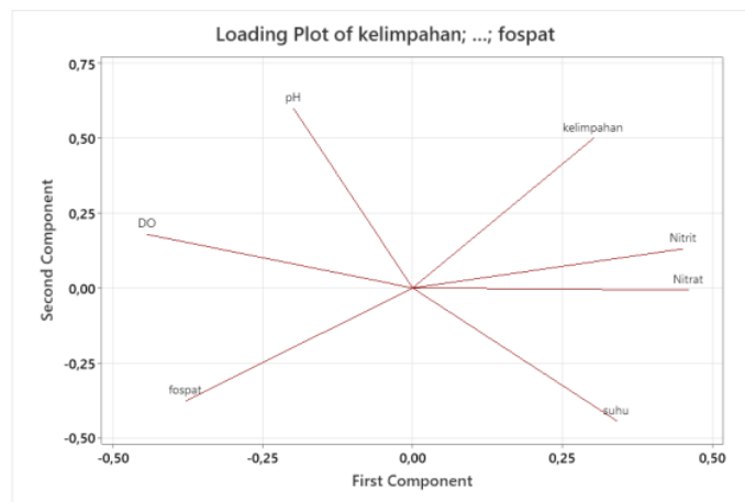
Gambar 4. 6 hubungan kelimpahan dengan parameter kualitas air
