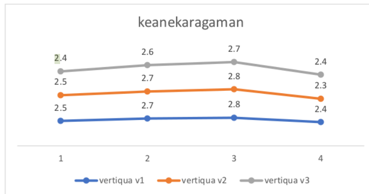
Gambar 4. 3 Grafik keanekaragaman fitoplankton
