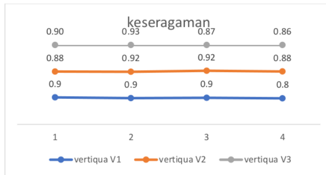
Gambar 4. 4 grafik indeks keseragaman
