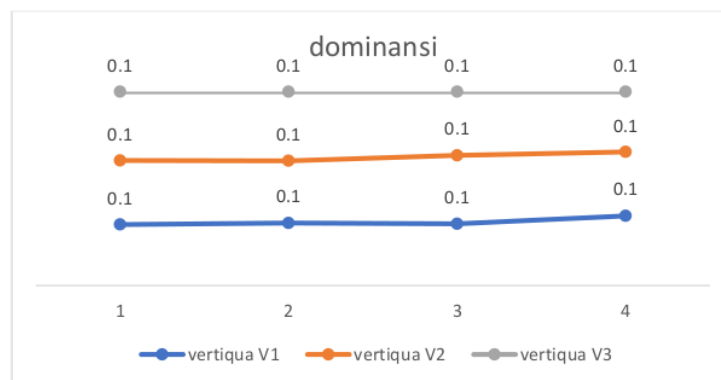
Gambar 4. 5 grafik indeks dominansi
